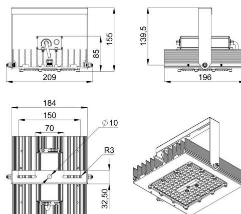
Габаритный чертеж
