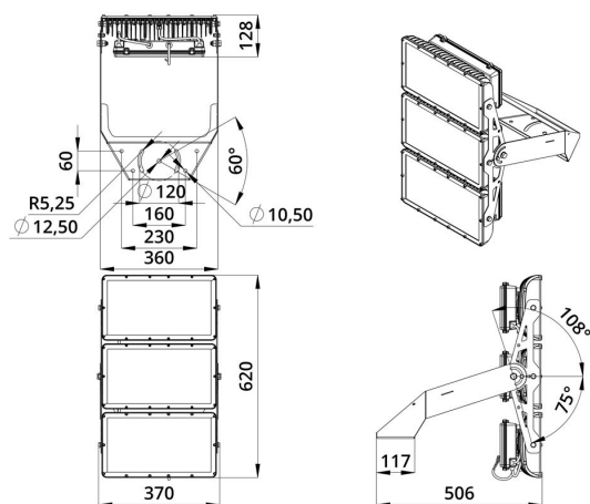
Габаритный чертеж
