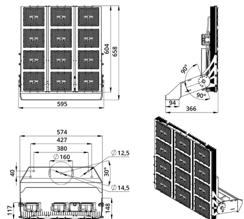
Габаритный чертеж
