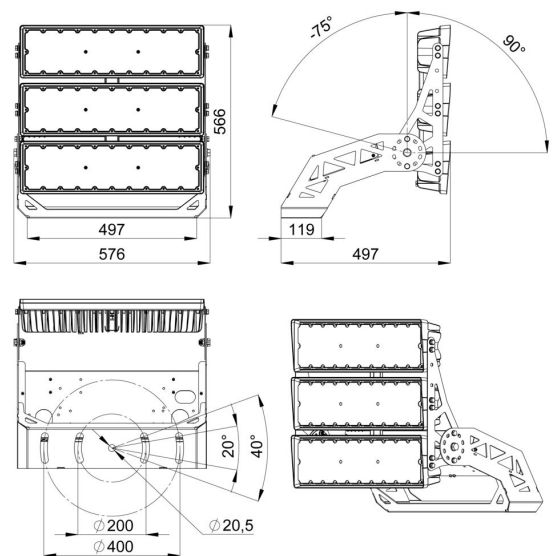
Габаритный чертеж
