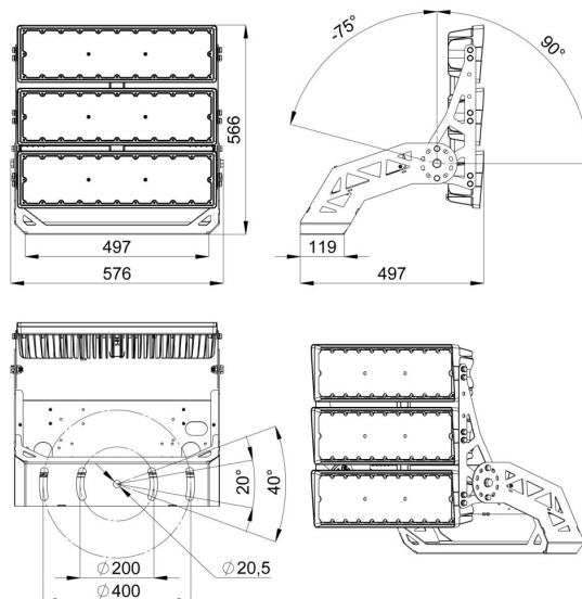
Габаритный чертеж
