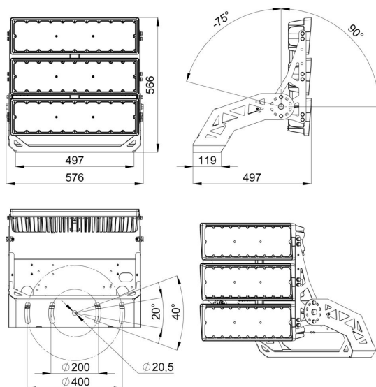
Габаритный чертеж
