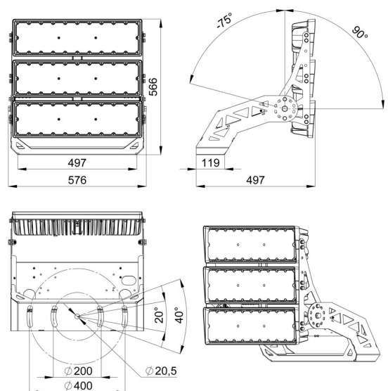
Габаритный чертеж
