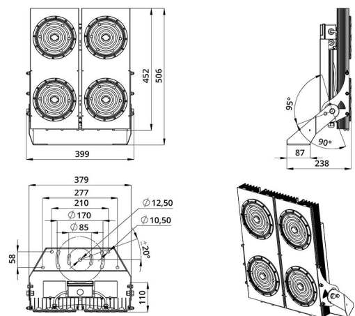
Габаритный чертеж
