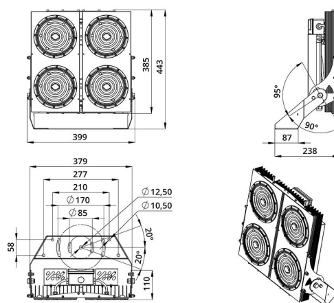
Габаритный чертеж
