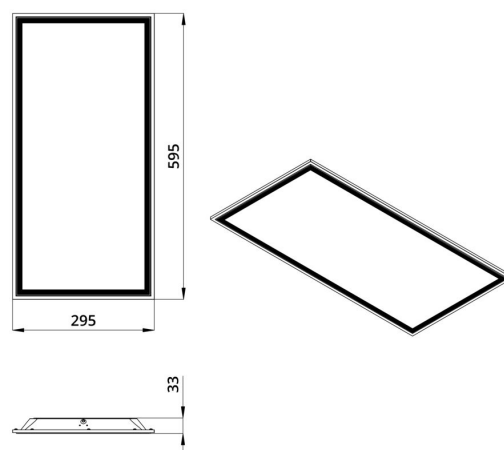
Габаритный чертеж
