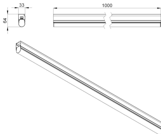
Габаритный чертеж
