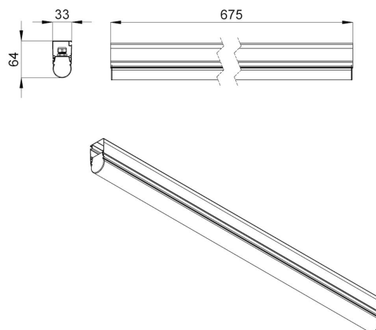
Габаритный чертеж
