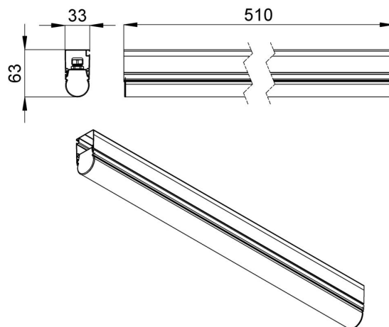
Габаритный чертеж
