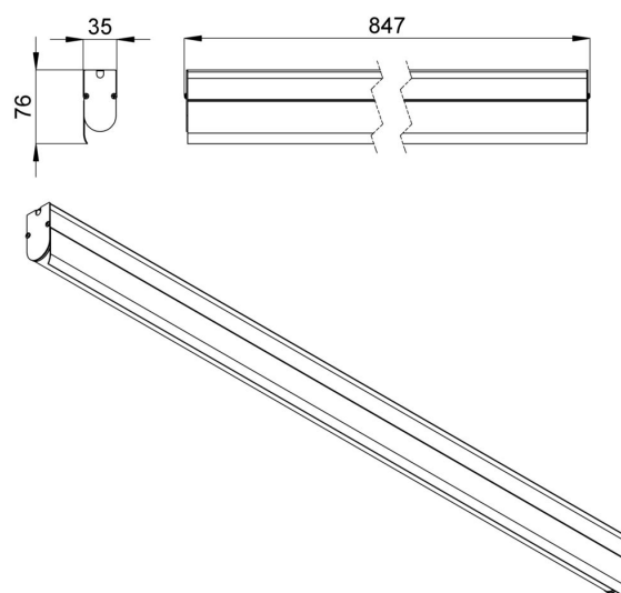
Габаритный чертеж
