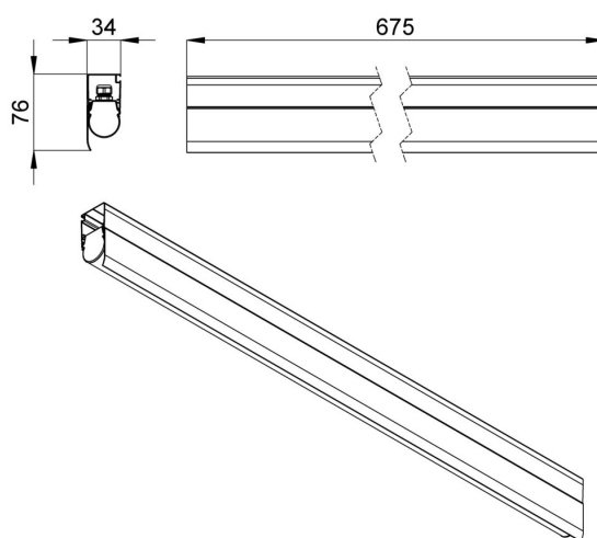
Габаритный чертеж
