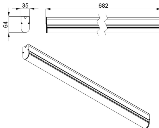
Габаритный чертеж
