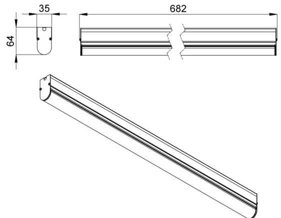
Габаритный чертеж
