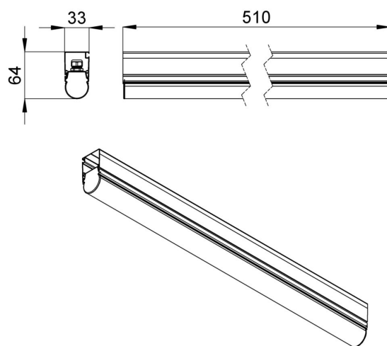
Габаритный чертеж
