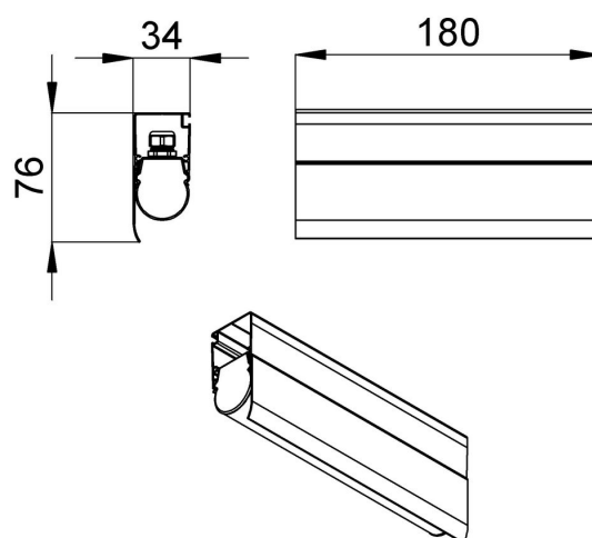
Габаритный чертеж
