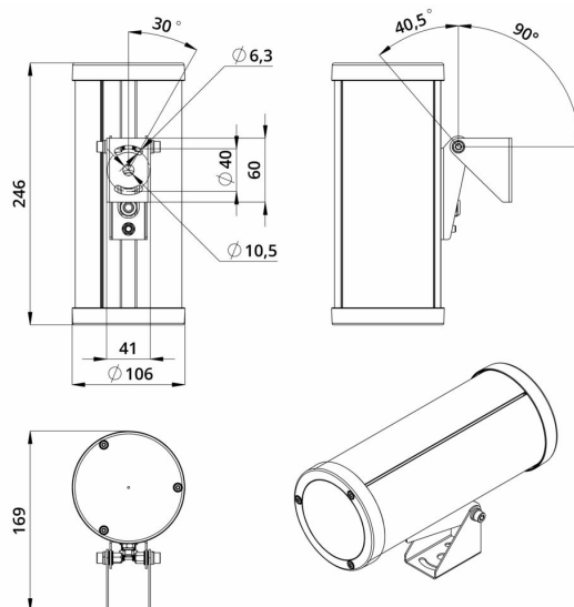
Габаритный чертеж
