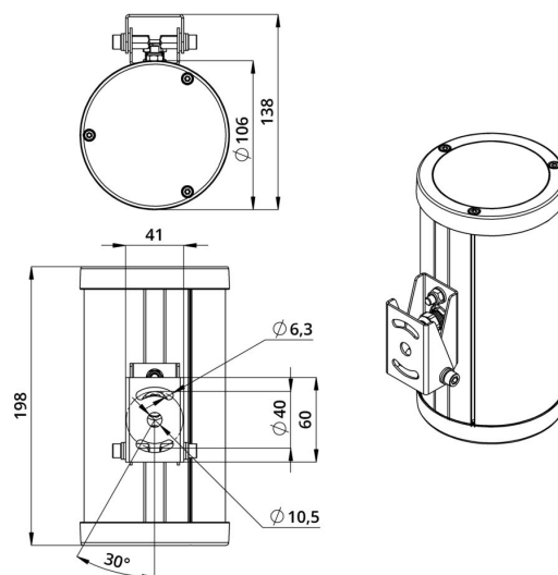
Габаритный чертеж
